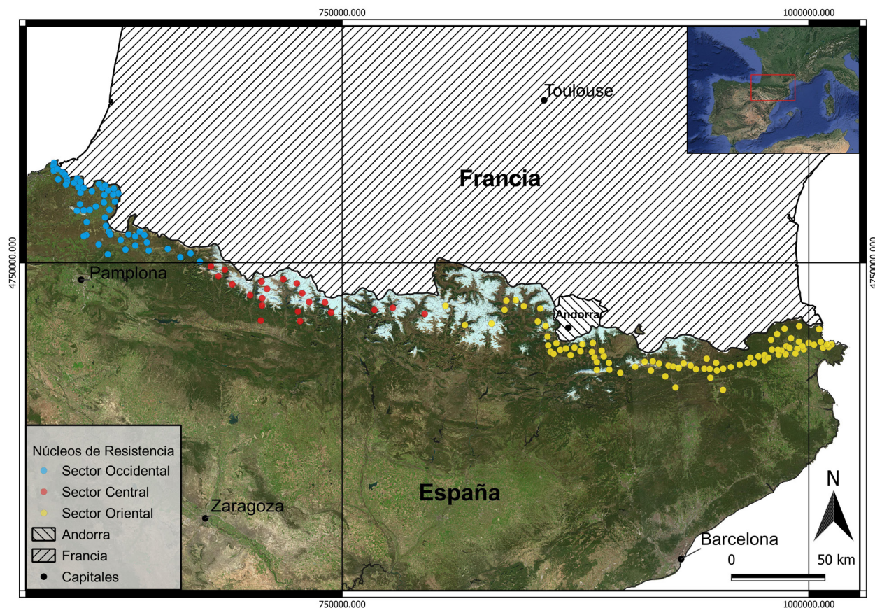
FIG. 4. Distribución de los núcleos de resistencia a lo largo del Pirineo divididos en tres sectores. Se aprecia la menor concentración de fortificaciones en las zonas de alta montaña. Reelaboración de Gabriel Alonso Díaz y el autor en base al diseño de P. Serrat, 1996.
