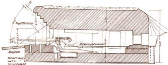
Schnitt A-B
