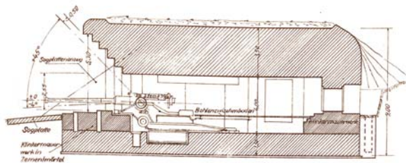
Schnitt A-B
