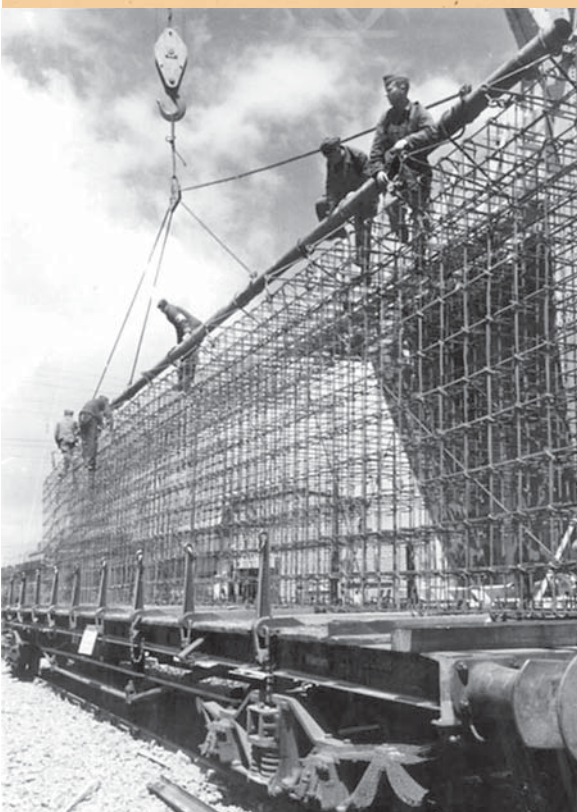
1943. Construcción del Muro Atlántico. Transporte de malla de hierro para construcción de búnkeres.
